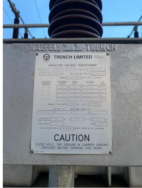
รูปที่ 1 VT 115 kV เฟส B ผลิตภัณท์ TRENCH ที่ สถานีไฟฟ้านครปฐม 2
